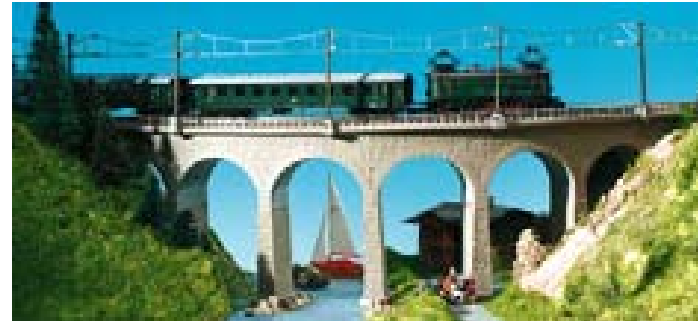
B-7665 Albulaviadukt ca. 31 x 3,8 x 10,1 cm Fahrbahnhöhe, mit Eisbrecher-Fundamenten, zwei- gleisiger Aufbau mit B-7664 möglich. Viaduktteile auch einzeln verwendbar. Radius 2=220-228,5 mm, ca. 90° – Albula Viaduct with ice breaker projections . Double track construction is possible when use with B-7664. Viaduct parts can also be used sepa- rately. R2 = 220-228,5 mm, 90°
