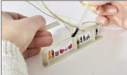
4. Die Füllstücke und die LED mit Kunststofffassung werden punktgenau über den Fenstern und Türen positioniert.
