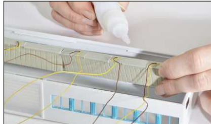
5. Dann wird die Lichtschiene hinter der Fensterreihe angeklebt.
