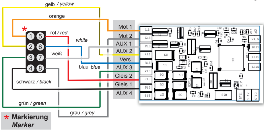
Abb. 3 Anschlusschema / Wiring connections
