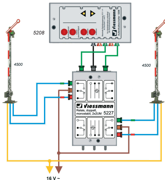
Abb. 3 Anschluss von Formsignalen am Aufenthaltsschalter 5208 Wiring of semaphore signals to the timer module 5208
